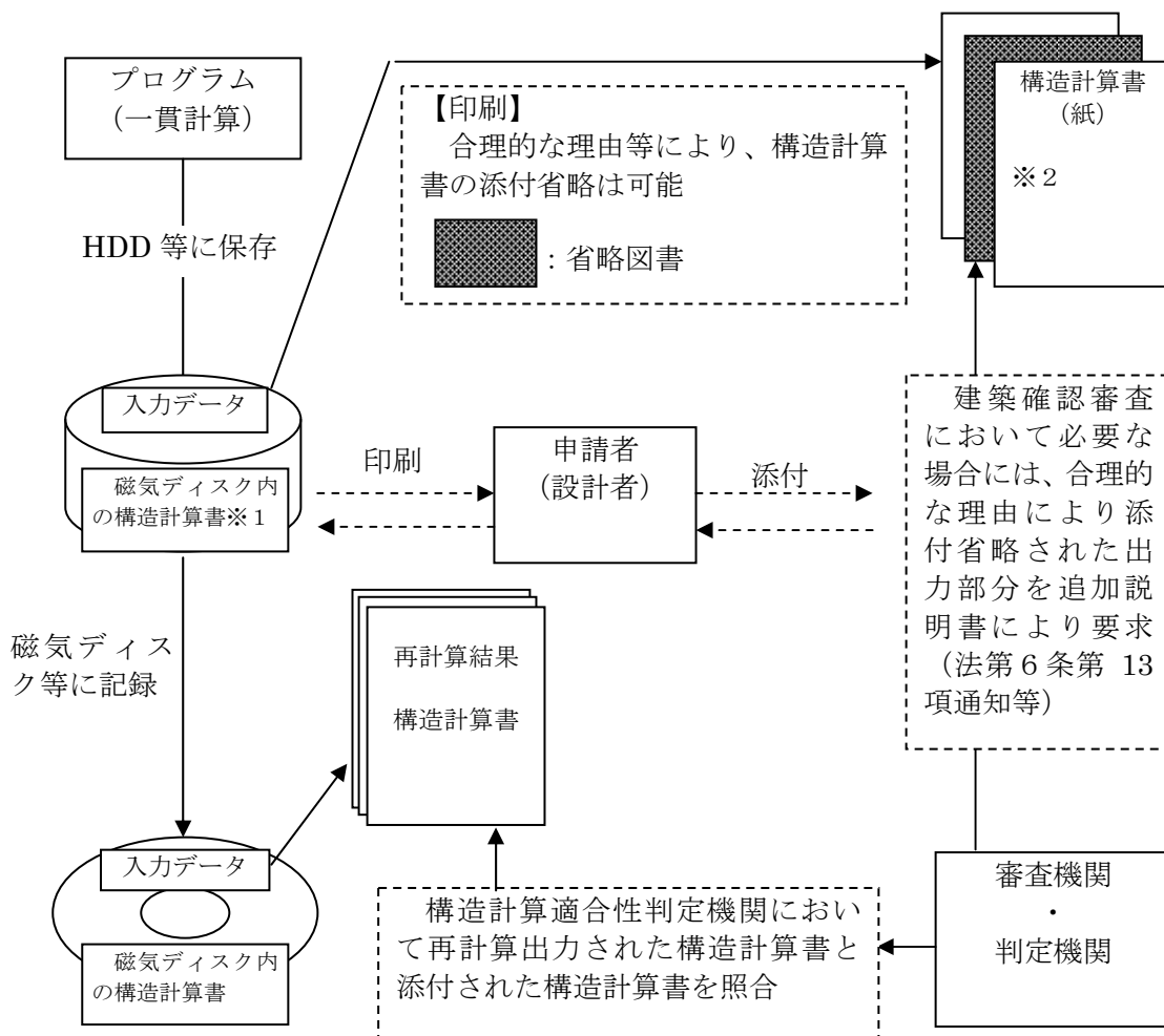
図 2.5-1 大臣認定構造計算プログラムによる構造計算書作成のフロー
