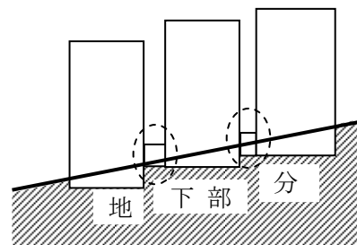
b) 地下部分と地上部分が水平方向に接続するもの
