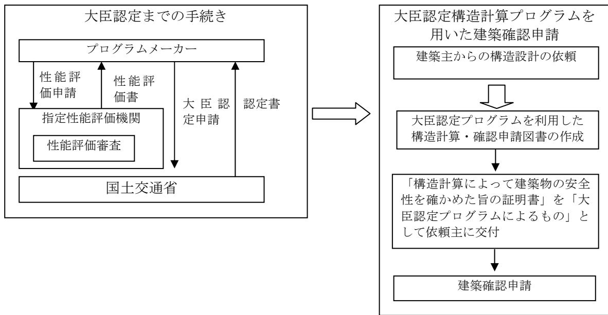
図 1.1-1 大臣認定構造計算プログラムの手続きと建築確認申請の流れ
