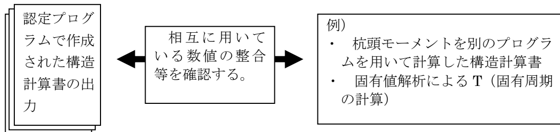
図 2.5-4 大臣認定構造計算プログラム以外のプログラム等を用いた場合の構造計算の審査
